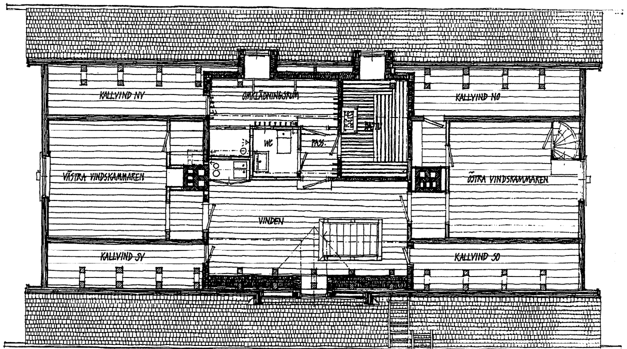
Lämningskåstället på Andholmen i Rönne OMRÖMNING: 1994. VINDPLAN. SKALA 1:50 23 februari 1994, Jan Wikström, arkitekt SAR 2
