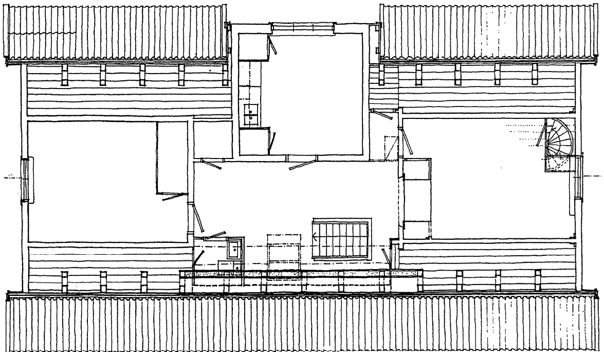
Lämningskåstället på Andholmen i Rönne UPPVÄRMNING. VINDPLAN. SKALA 1:50 15 november 1993, Jan Wikström, ark. SAR 10
